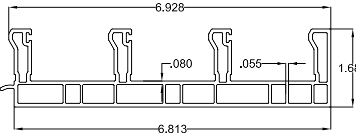
1B FRAME - 3T
