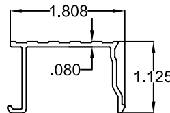
6 SILL CAP
