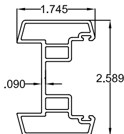
40 ASTRAGAL
