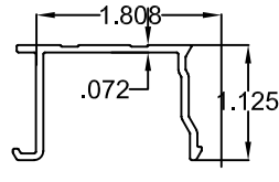
4 FRAME CAP
